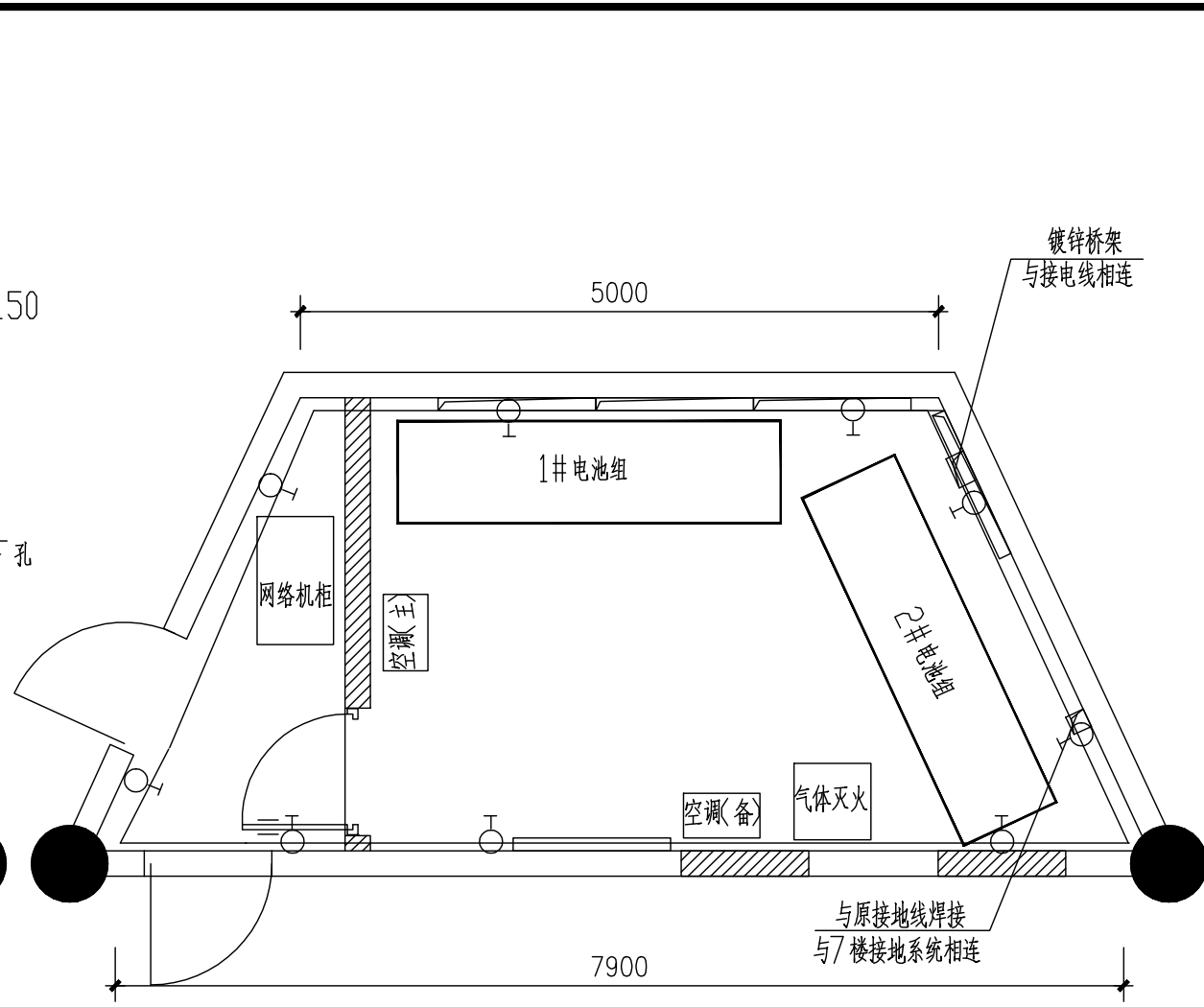
裙房6F 电池间接地平面图 1:50
