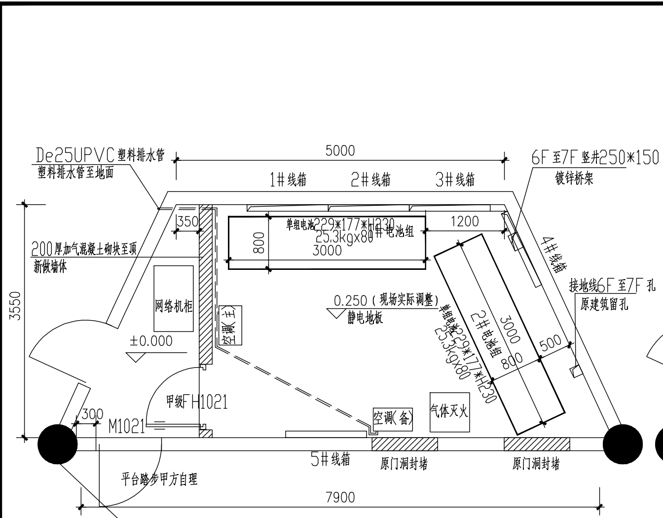
裙房6F 电池间平面布置图 1:50
